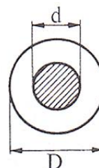
Rys. 7.1.3. Wymiary kabla
