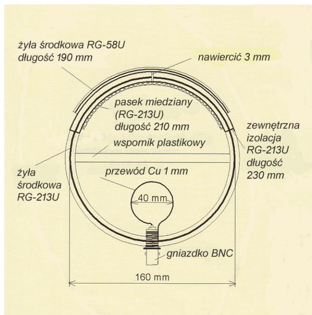
Rys. 6.2.1. Konstrukcja anteny Fot. 6.2.2. Widok gotowej anteny
