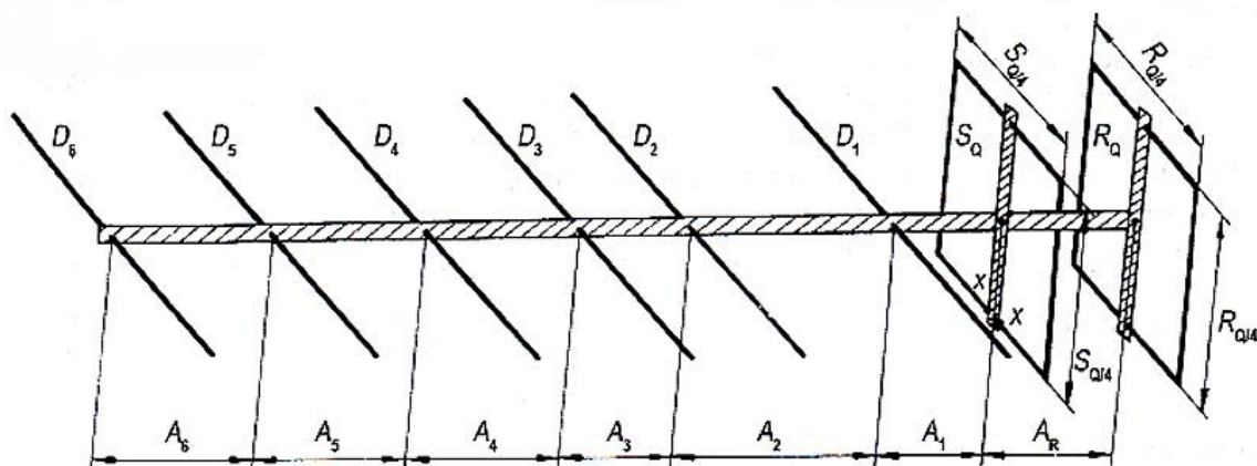
Rys. 3.1.2. Antena ósmioelementowa. Wymiary podano w tabeli 3.1.1
