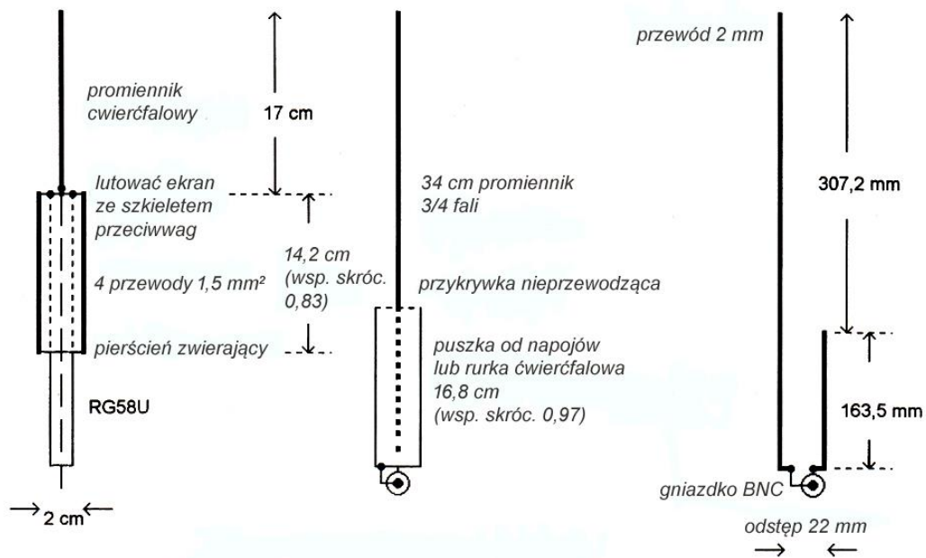
Rys. 4.3.3. Porównanie konstrukcji
