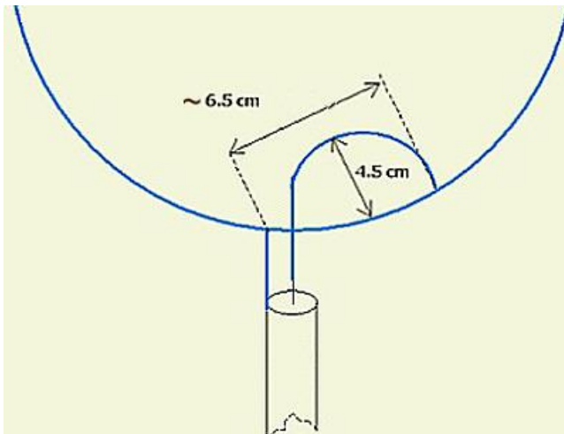
Rys. 6.3.1. Konstrukcja anteny ósemkowej na 145 MHz Rys. 6.3.2. Transformator półkolisty
