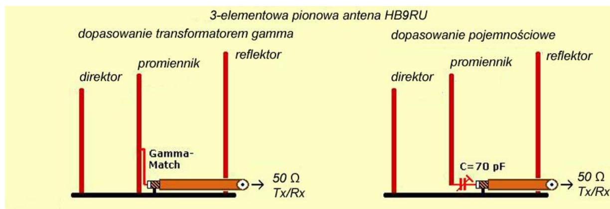
Rys. 4.1.1. Konstrukcja i warianty zasilania anteny HB9RU a – transformator gamma, b – kondensator szeregowy
