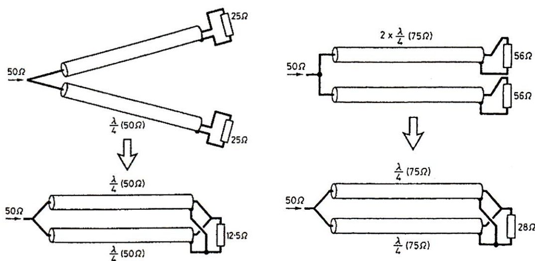
Rys. 7.5.1. Dopasowanie oporności 12,5 \Omega za pomocą dwóch odcinków 50-omowych
