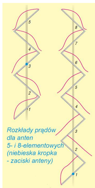
Rys. 5.5.2. Rozkłady prądów
