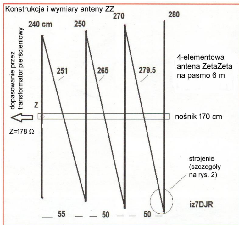
Rys. 5.5.6. Konstrukcja anteny ZZ
