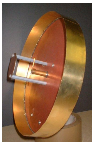
Rys. 2.2.3. Przykład realizacji anteny na pasmo 2,4 GHz
