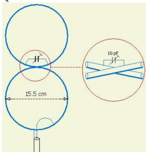
Rys. 6.3.1. Konstrukcja anteny ósemkowej na 145 MHz Rys. 6.3.2. Transformator półkolisty
