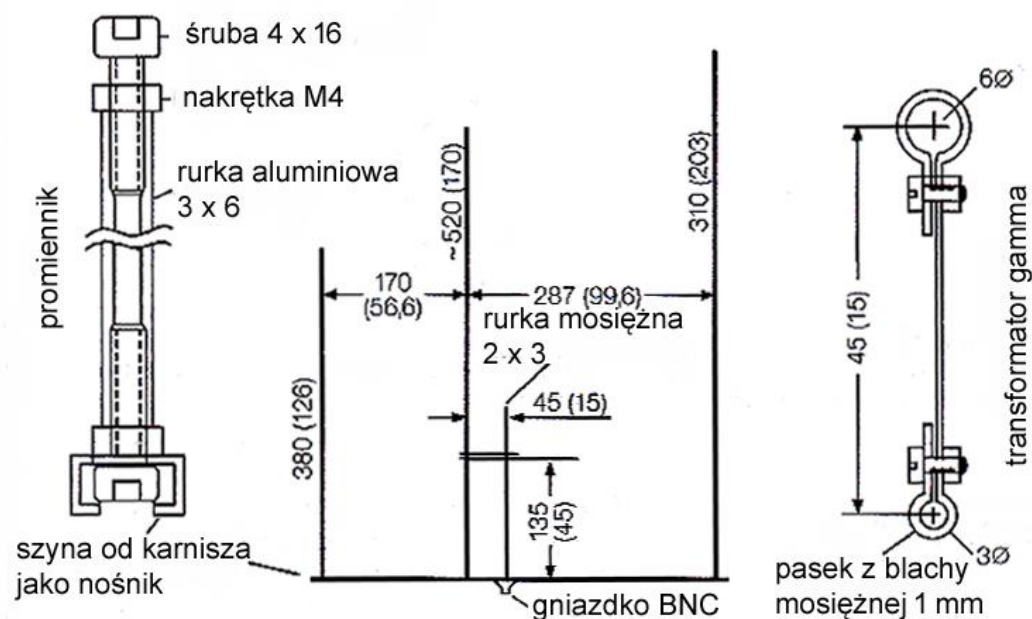
Rys. 4.1.2. Antena HB9RU na pasma 2 m i 70 cm (wymiarzy w nawiasach)
