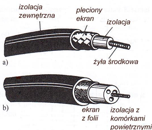
Konstrukcje kabli współosiowych
