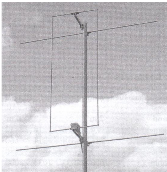
Rys. 3.2.1. Konstrukcja anteny i oznaczenia elementów. Przy zasilaniu poziomego boku jak na rysunku antena ma polaryzację poziomą
