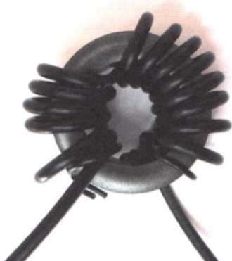
Fot. 3.4.6. Wykonanie dławika fali powierzchniowej z kabla RG174
