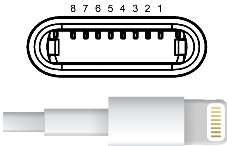
Rys. 2.1.1. Gniazdko i wtyczka „Lighting”
