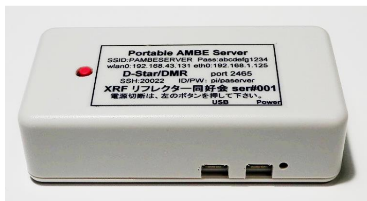
Fot. 1.3.8. Portable AMBE Server składa się z Maliny z dodaną płytką wokodera
