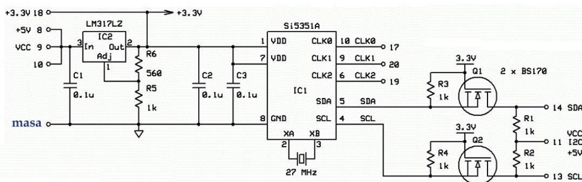
Rys. 3.2.1. Schemat ideowy generatora sygnałowego
