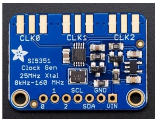
Fot. 3.2.3a. Moduł Si5351A firmy Adafruit Rys.3.2.3b. Schemat blokowy Si5351A. Zawiera on dwa synchronizowane fazowo generatory VCO (PLL A i PLLB) pracujące w zakresie 600 – 900 MHz i programowalne dzielniki pozwalające na uzyskanie ułamkowych stosunków podziału i w ten sposób pożądanych częstotliwości wyjściowych
