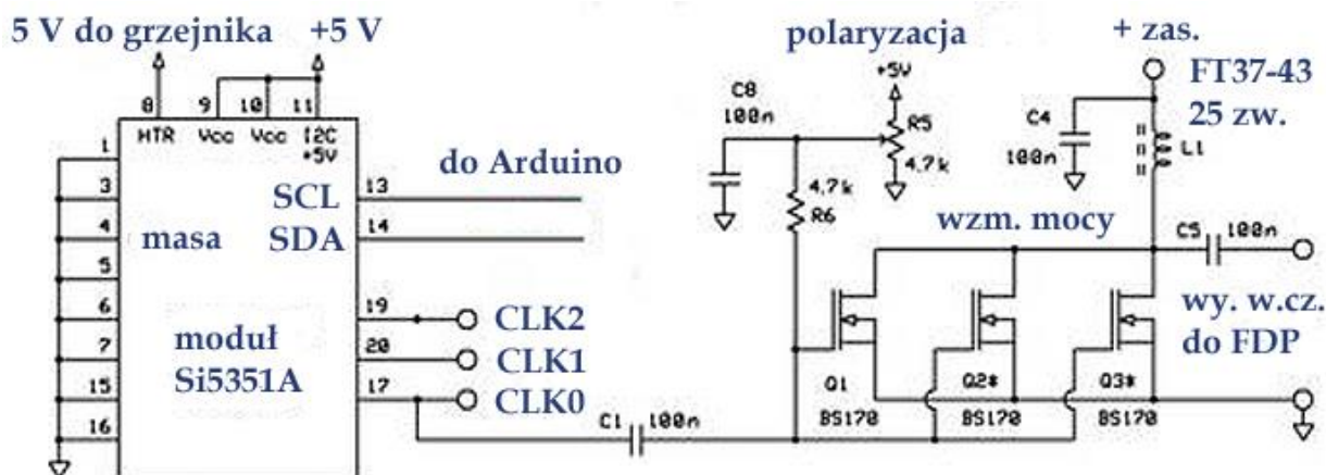
Rys. 3.3.2.4. Schemat toru w.cz. z modułem Si5351A w TCXO
