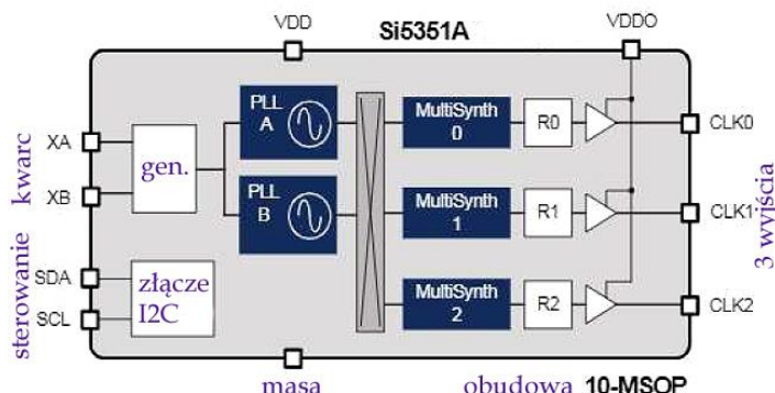
Fot. 3.2.3a. Moduł Si5351A firmy Adafruit Rys.3.2.3b. Schemat blokowy Si5351A. Zawiera on dwa synchronizowane fazowo generatory VCO (PLL A i PLLB) pracujące w zakresie 600 – 900 MHz i programowalne dzielniki pozwalające na uzyskanie ułamkowych stosunków podziału i w ten sposób pożądanych częstotliwości wyjściowych
