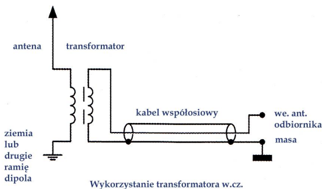
Rys. 3.4.5. Schemat podłączenia
