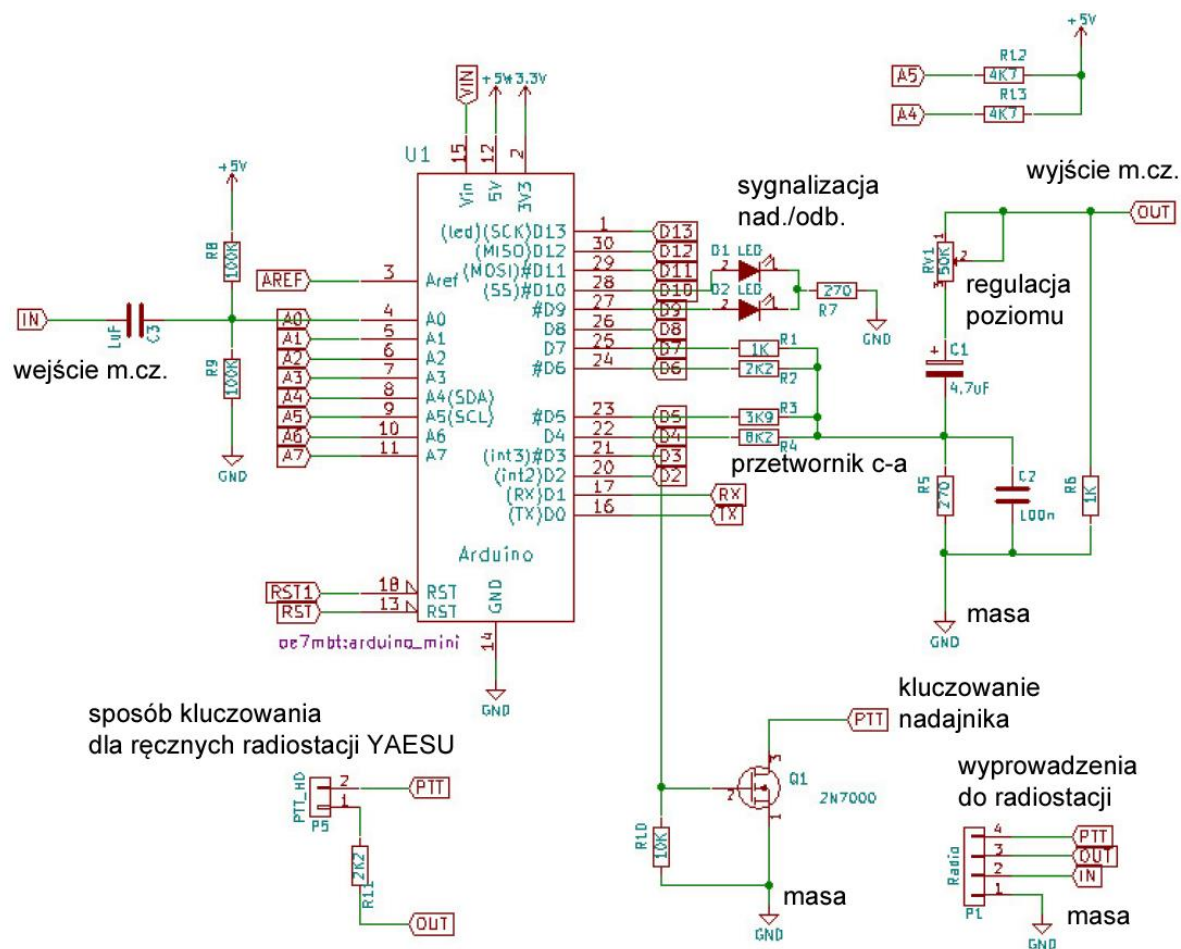
Rys. 3.1.2.1. Schemat ideowy modemu
