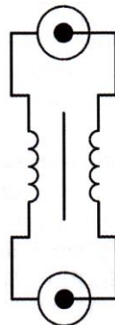
Fot. 3.4.6. Wykonanie dławika fali powierzchniowej z kabla RG174
