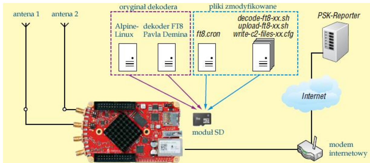
Rys. 8.2. Schemat blokowy współpracy „Red Pitayi” z dwoma antenami i serwerem PSK-Reporter w Internecie. Pliki w niebieskiej ramce są do pobrania z witryny Funkamateura , we fioletowej są częścią rozwiązania Pavla Demina
