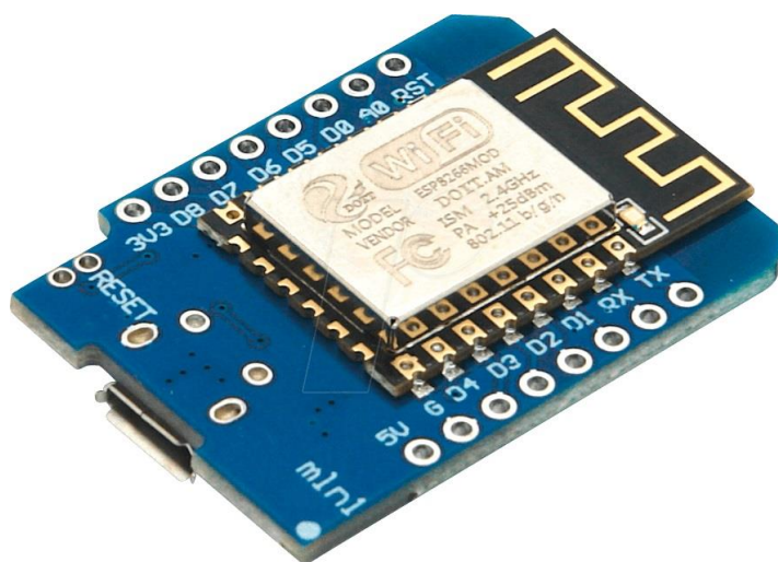
Fot. 4.2.5. Moduł D1 MINI ESP8266 użyty w nadajniku WB2CBA posiada 11 wyprowadzeń logicznych, złącza I2C i 1Wire, gniazdko USB, wyjście sygnału z modulacją szerokości impulsów, wejście analogowe 3,3 V i 4 MB pamięci programu, ale nie posiada złącza SPI i kieszeni dla pamięci SD
