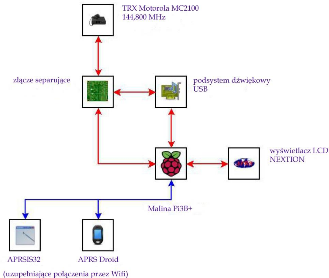
Rys. 5.6.1. Schemat blokowy stacji przekaznikowej SQ9MDD
