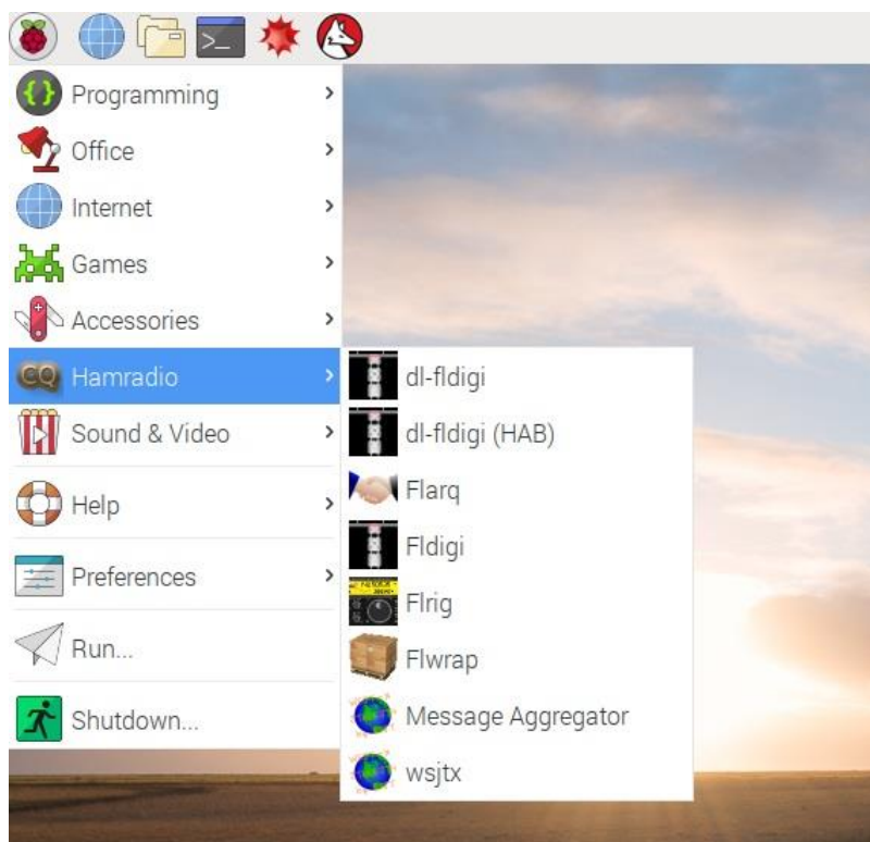
Rys. 5.3.2.2. Wywołanie WSJT-X
