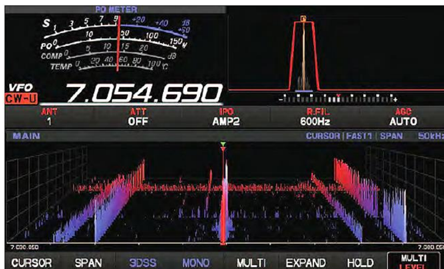
Fot. 1.2. Ten sam podzakres po włączeniu wskaźnika trójwymiarowego. Zastępuje on zwykły wskaźnik wodospadowy. Trzecim wymiarem jest czas, którego oś przebiega perspektywicznie w głąb wskaźnika.
